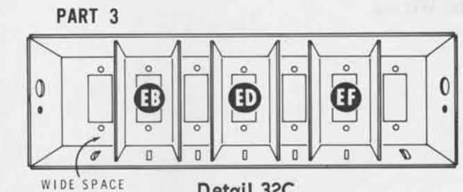
Detail 32C
