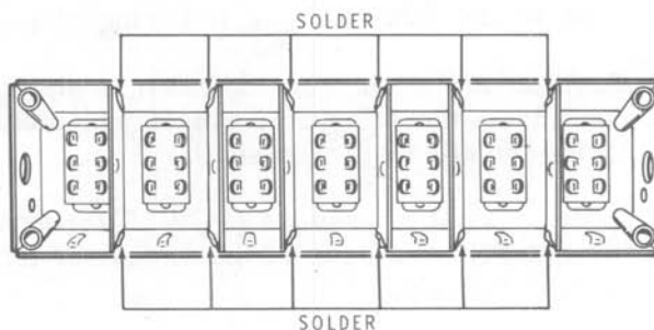
Detail 32E
